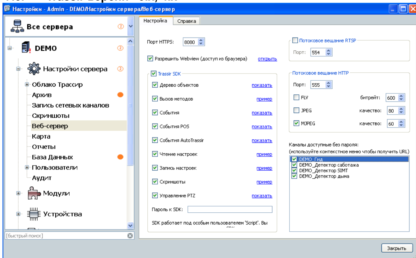
Рисунок 19. Настройки сервера системы видеонаблюдения Trassir 3.
