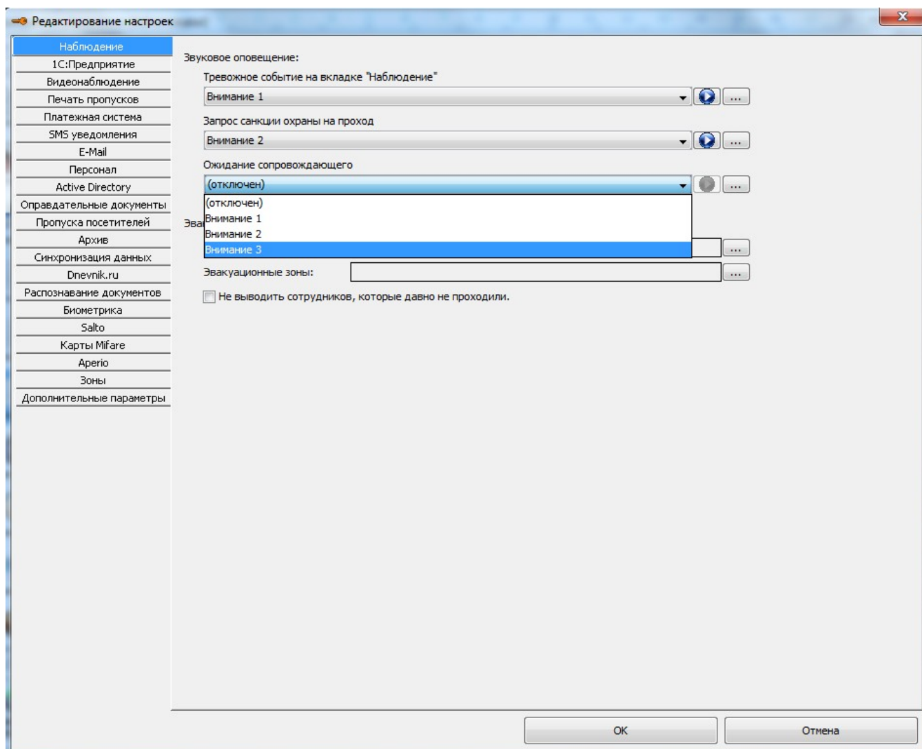
Рисунок 122. Настройки звуковых оповещений ПО «Наблюдение и фотоидентификация».
