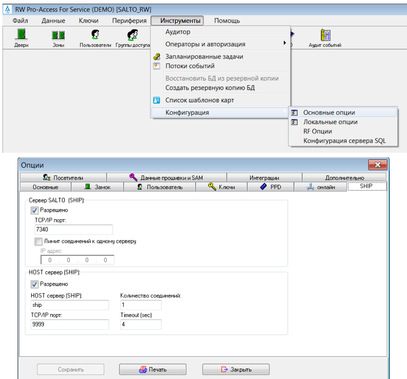
Рисунок 278. Настройка ship-протокола в Salto.
