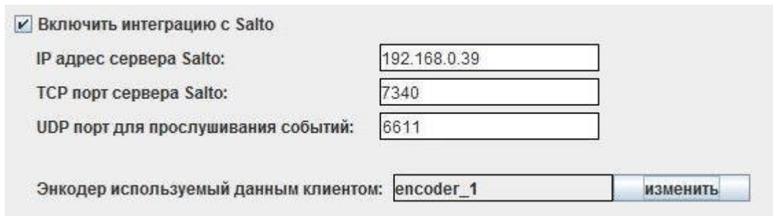
Рисунок 282. Настройка интеграции с Salto в СКУД Sigur.
