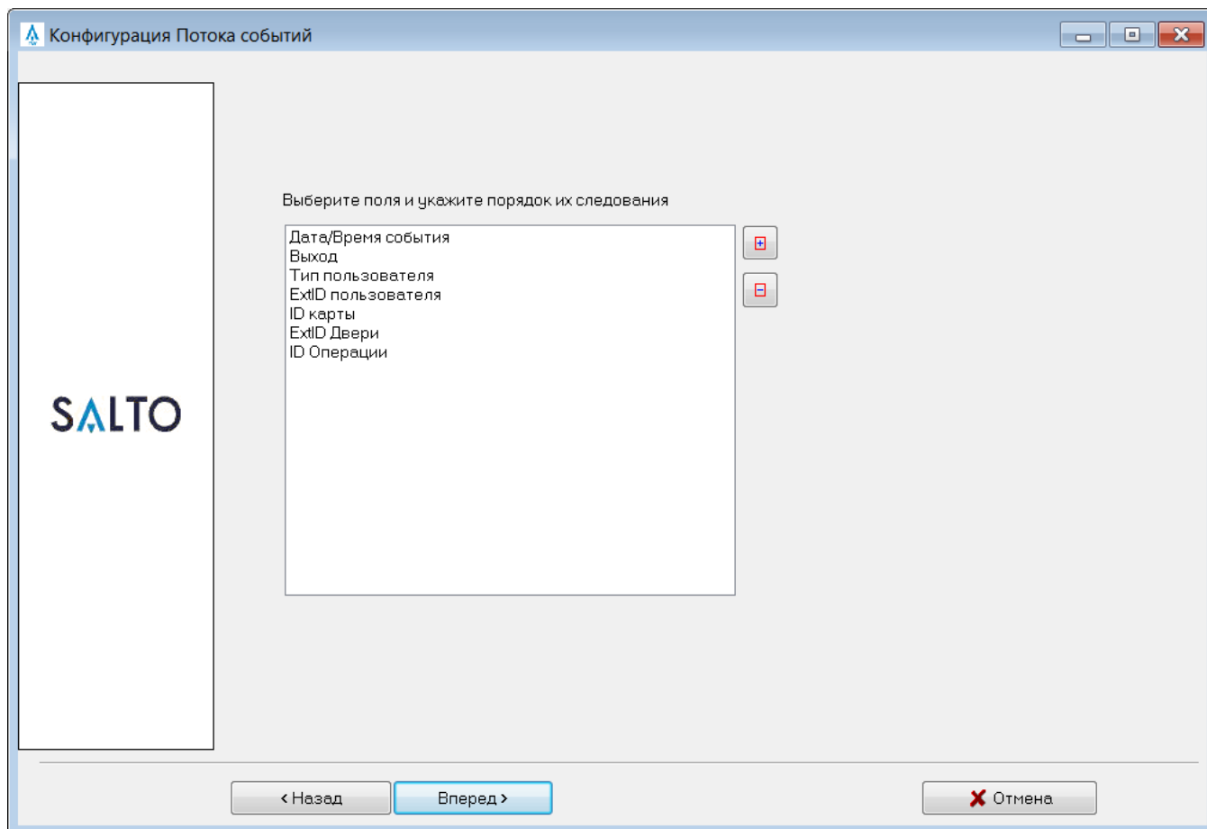
Рисунок 281. Выбор полей в конфигурации Потока событий в Salto.
