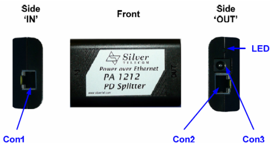
Рисунок Б.1 Внешний вид сплиттера
