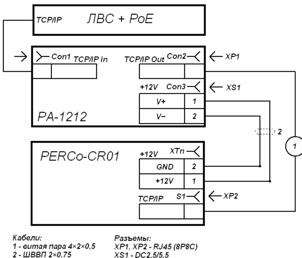
Рисунок Б.2 Схема подключения контроллера через PoE-сплиттер PA1212
