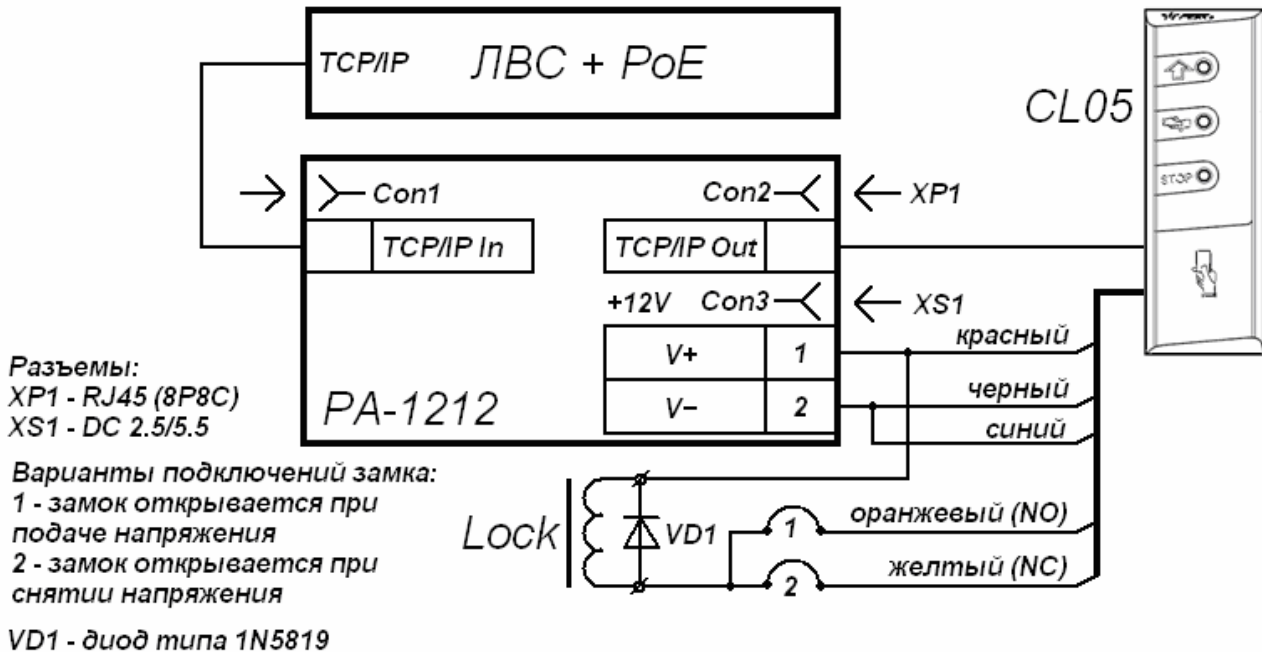
Рисунок В.2 Схема подключения контроллера через PoE-сплиттер PA1212 (Lock – замок, управляемый контроллером)
