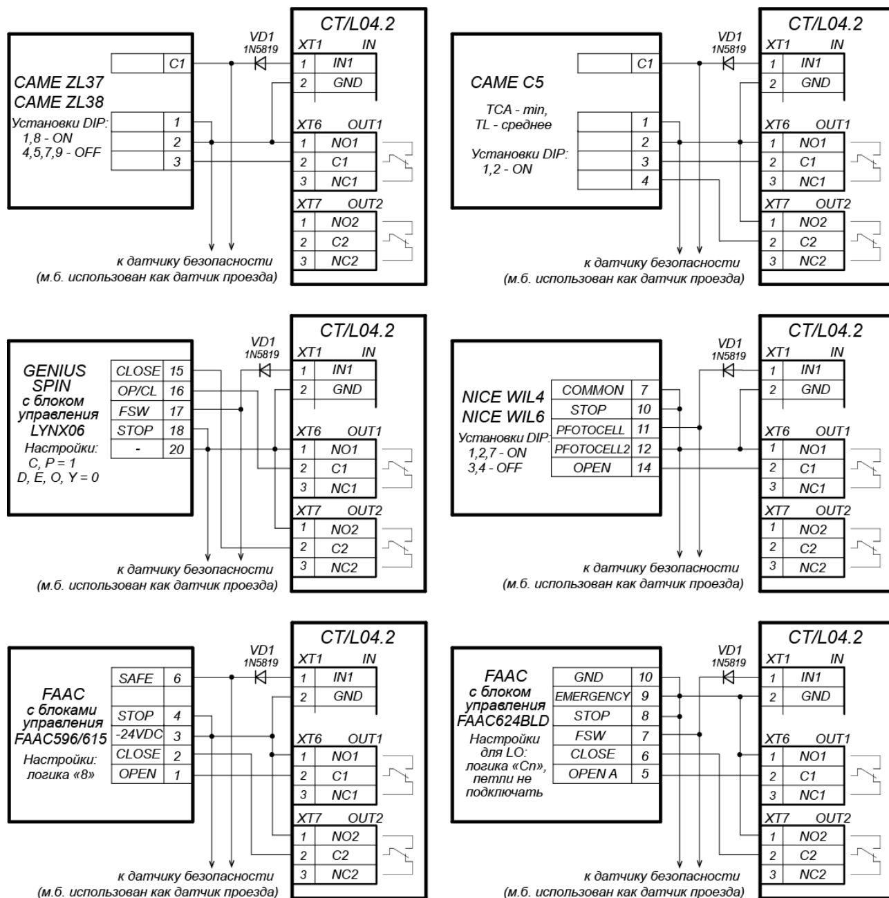
Рисунок 8. Примеры схем подключения шлагбаумов к контроллеру АТП
