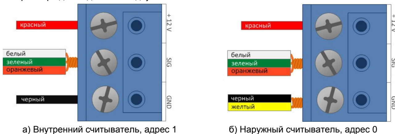
Рисунок 4. Подключение считывателя в режиме Parsec
