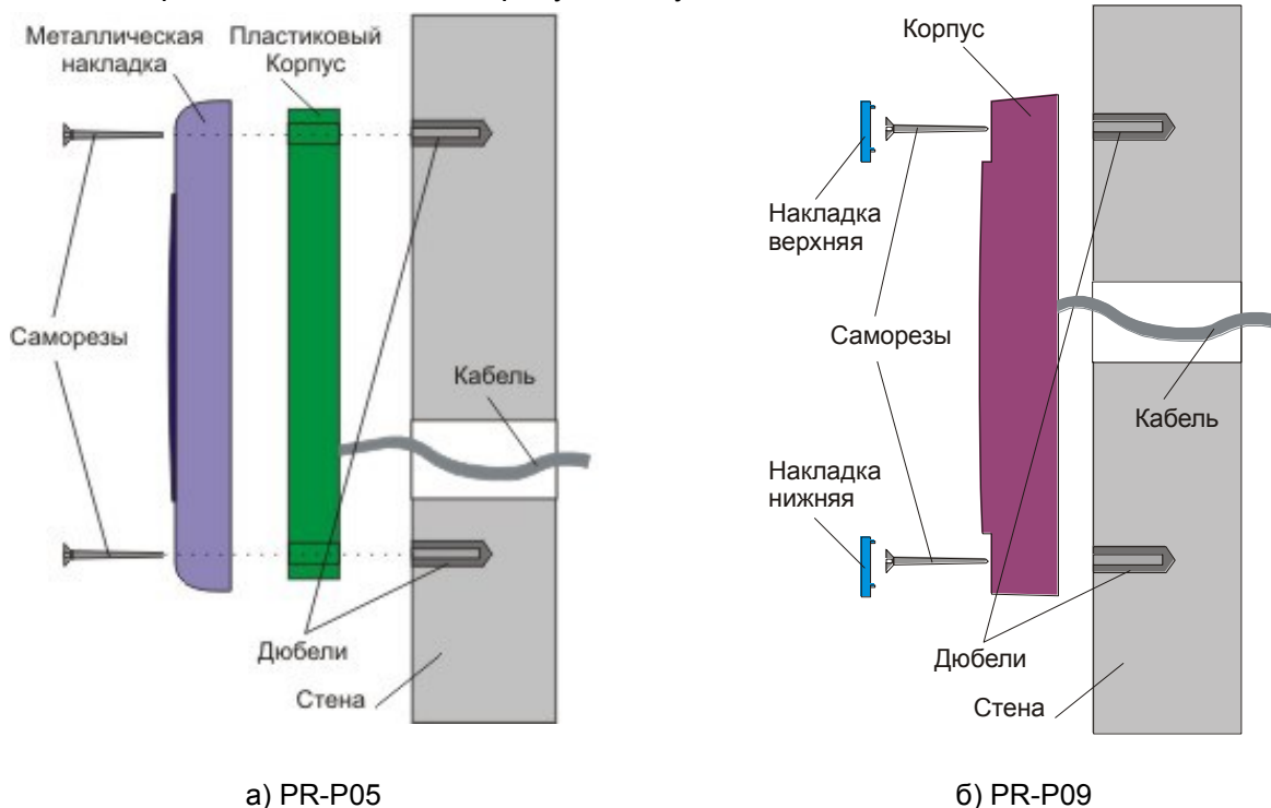
Рисунок 2. Крепление считывателей
