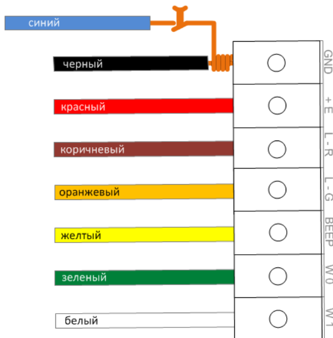
Рисунок 6. Включение защищенного режима при подключении по Wiegand 26
