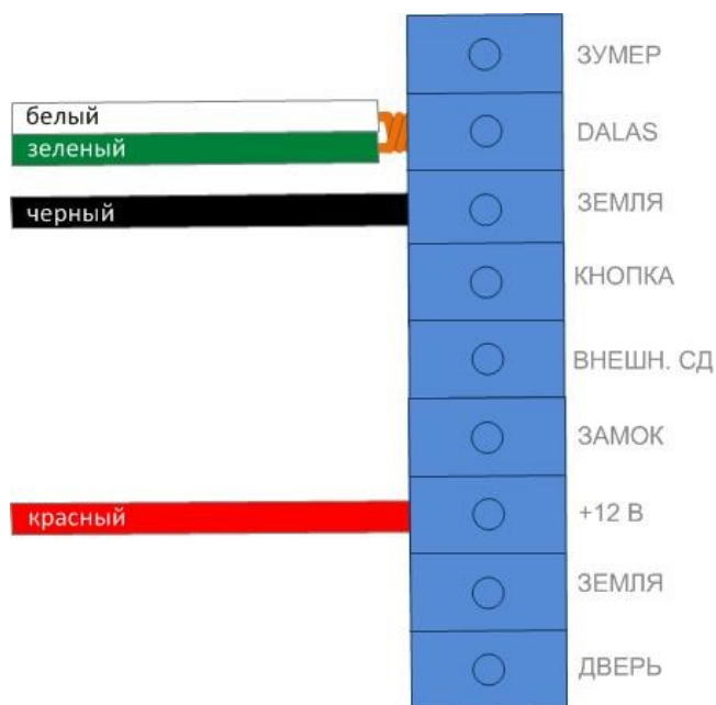
Рисунок 3. Пример подключения считывателя в режиме Touch Memory
