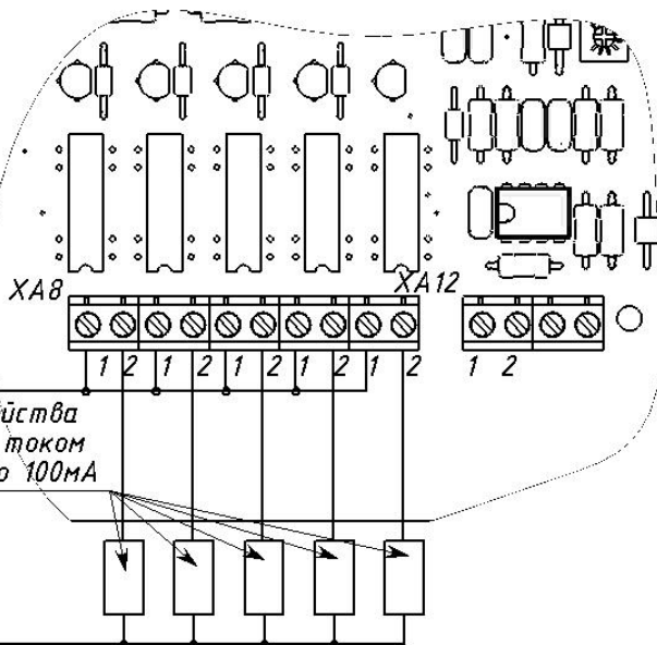
Рисунок 5 – Подключение внешних устройств автоматики.
