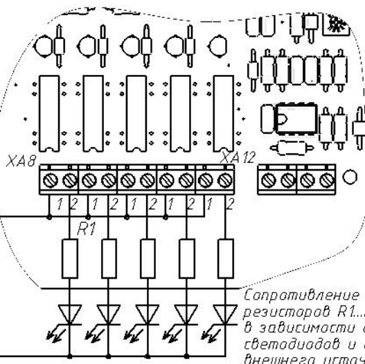
Рисунок 6 – Подключение внешних индикаторов
